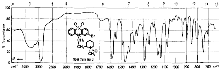
Fig. 3. IR.-Spektrum der Base des 3-Brom-10-{2'-[N-methylpiperidyl-(2'')]-äthyl-(1')}-phenothiazin-9-sulfon-N-oxydes in Nujol
